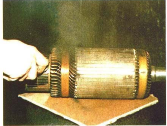
2) Anker wordt schoongeblazen met perslucht.
